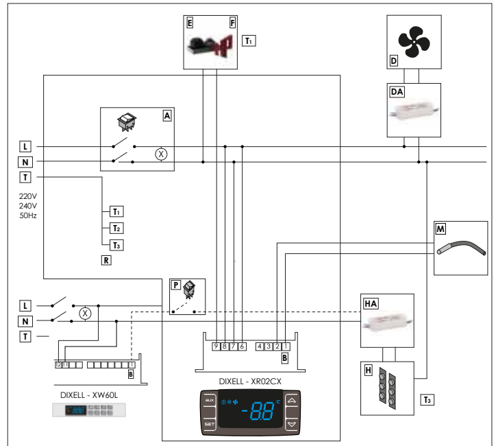
PM-VBR10 / PC-VBR10
